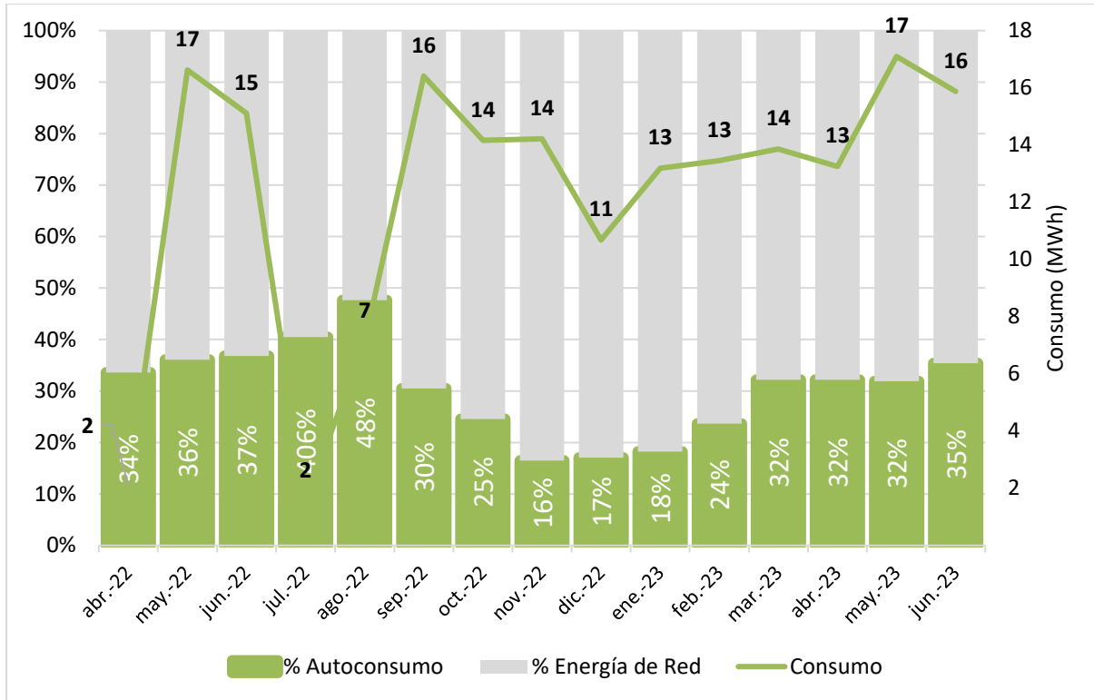
Figura 3: Consumo energético, % De autoconsumo y energía importada desde la instalación hasta la realización de la memoria por meses (Megapunt)
