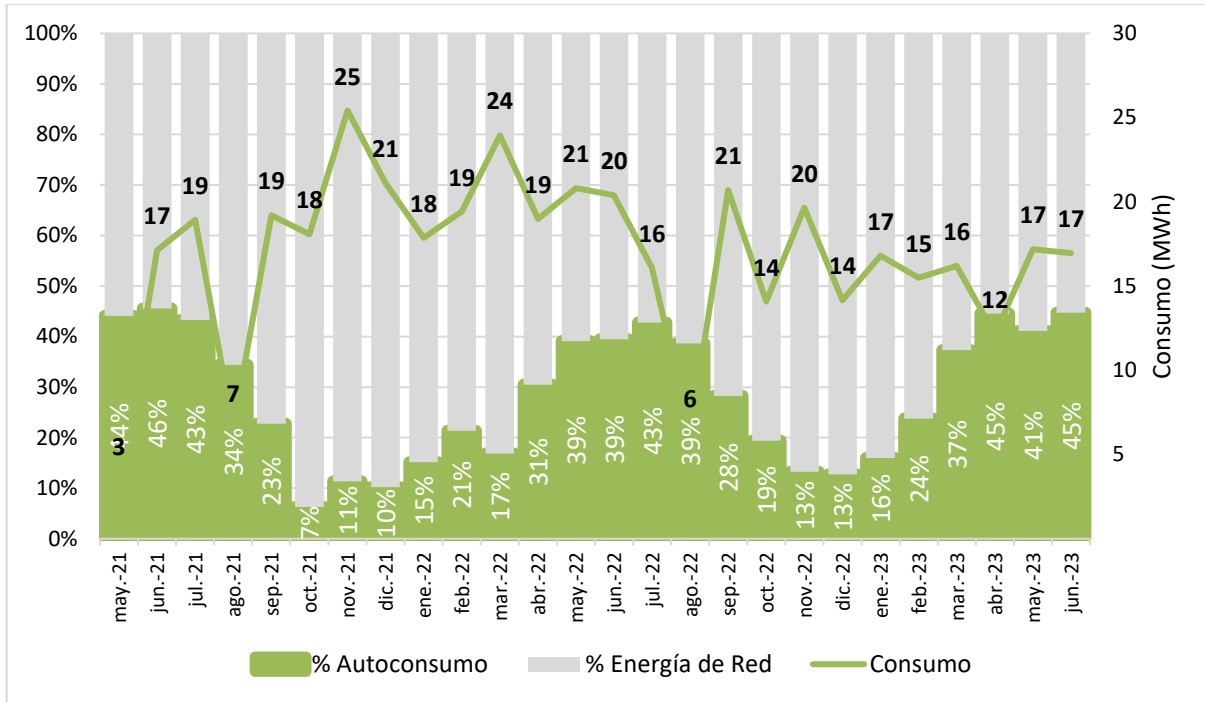
Figura 1: Consumo energético, % De autoconsumo y energía importada desde la instalación hasta la realización de la memoria por meses (Felper).
